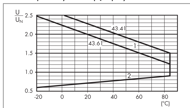
R 43 - DC Dopuszczalny zakres napięcia pracy cewki
